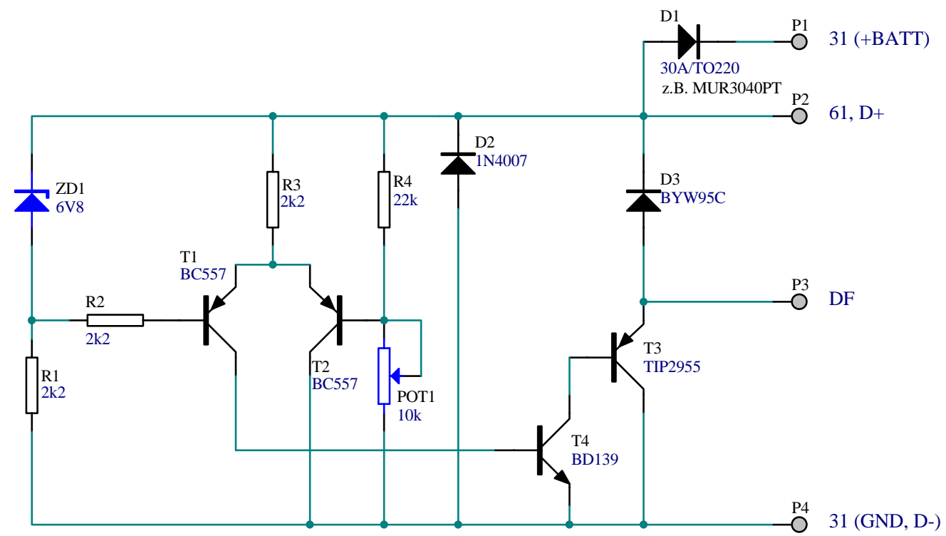
LiMa-Regler 6V
